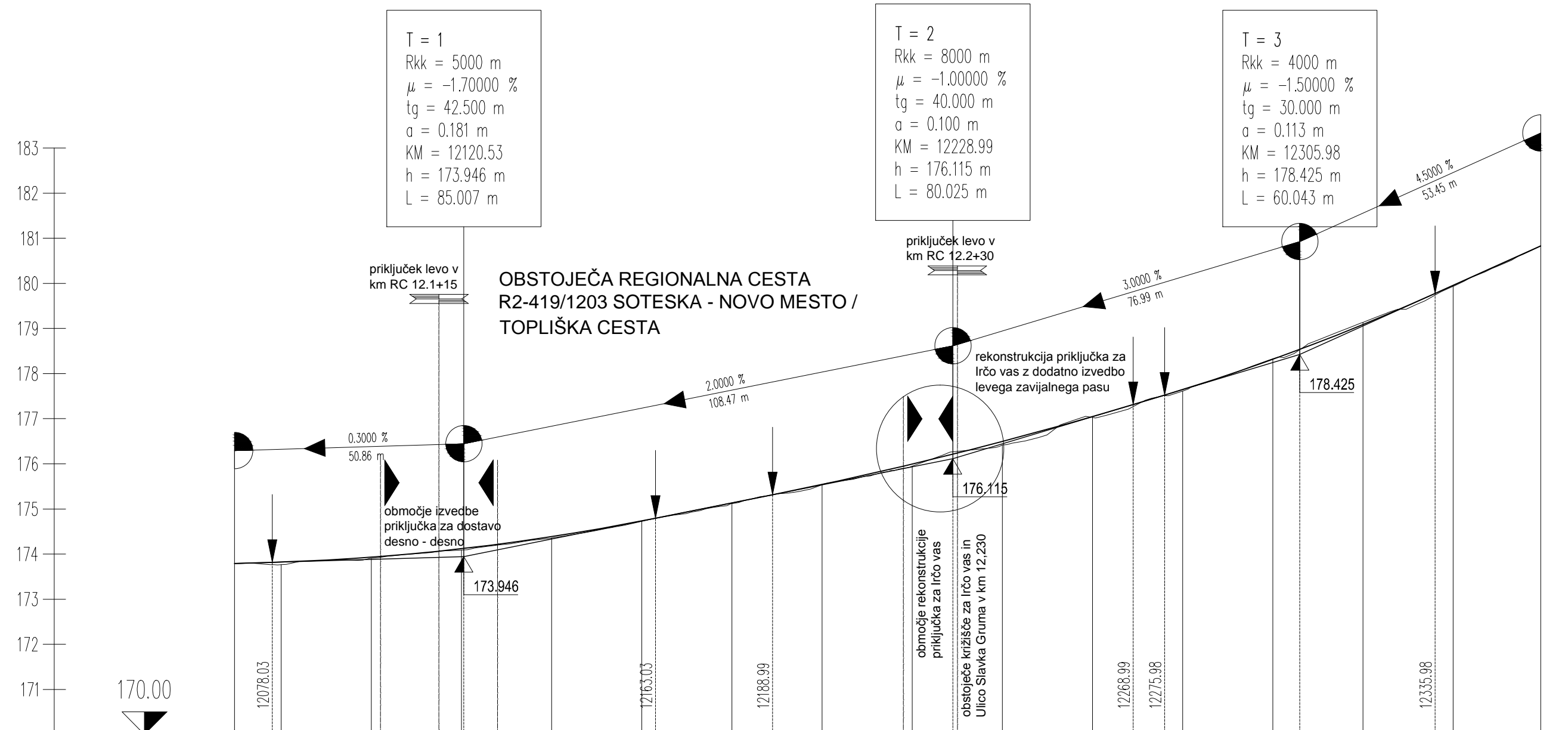
PROFIL-1: OS_REGIONALKA MERILO 1:1000/100
